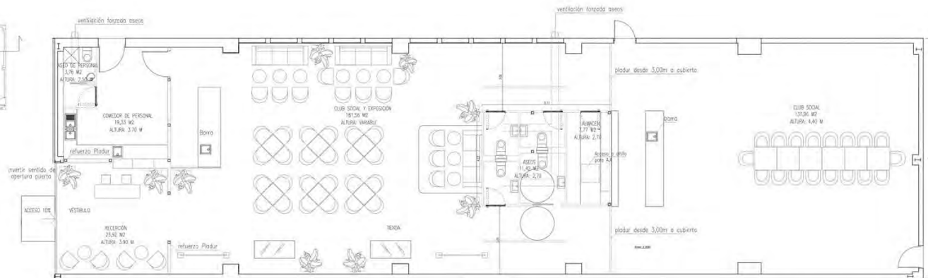
PLANTA NAVE
